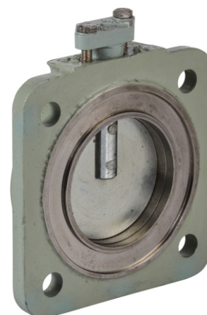
MODEL: CS80 G 211 (MS/SS bolt)
